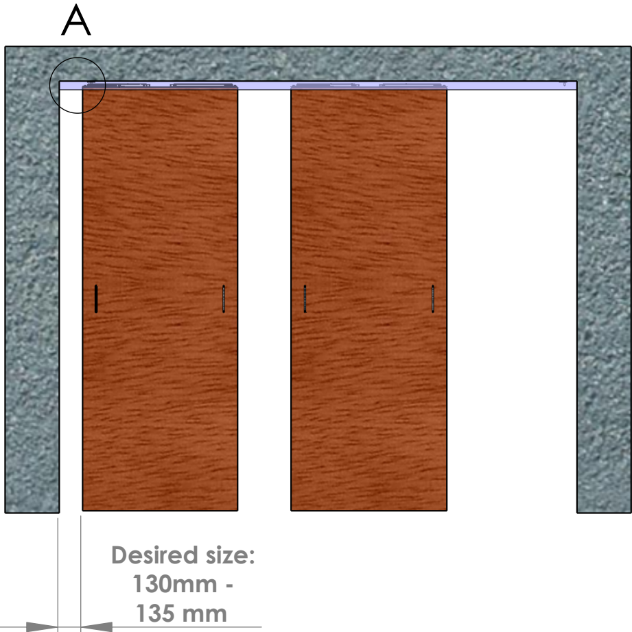
DETAIL A MAßSTAB 1 : 3
